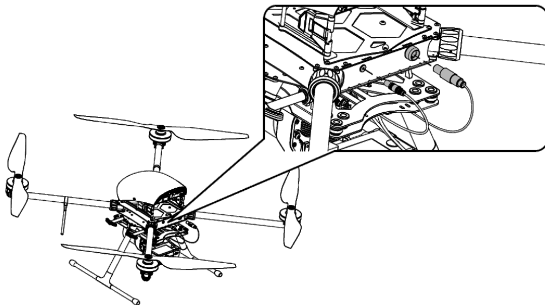
Подключение двух кабелей полезной нагрузки на примере лазерного сканера
