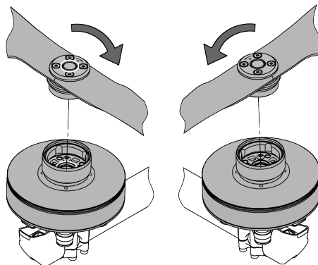
Установка быстросъемных винтов
