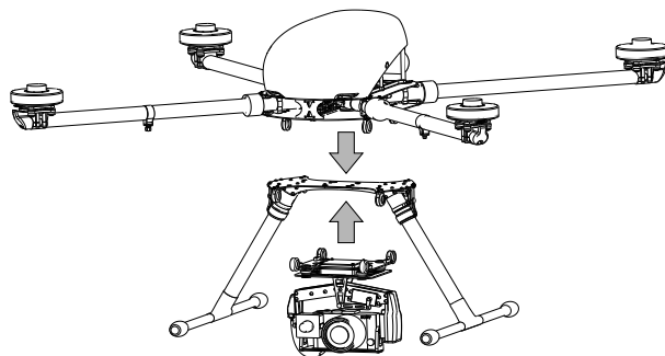
Пример установки квадрокоптера и подвеса камеры на шасси
