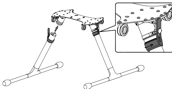
Установка и фиксация стоек шасси
