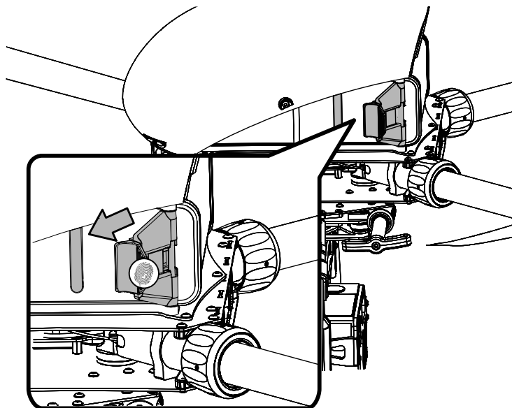
Фиксация АКБ подпружиненными упорами
