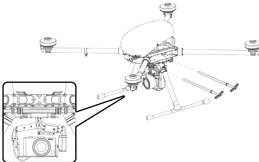
Установка соединительных штырей
