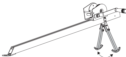
Установка опорных стоек задней части
