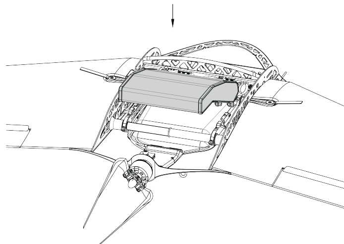
Установка АКБ
